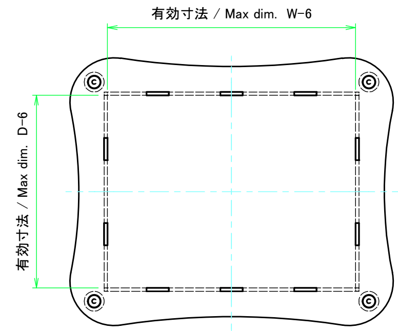
下カバー / Bottom cover
