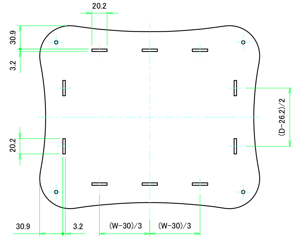
上カバー裏面 / Top cover Backside
