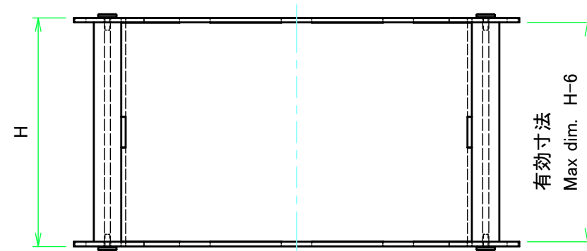
Wパネル1 / W panel 1
